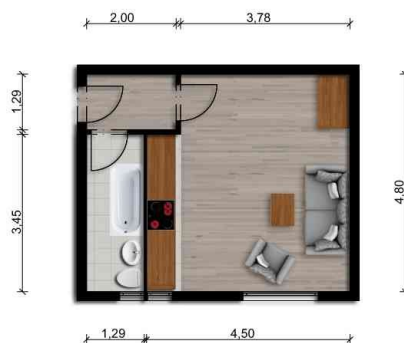
Grundriss
