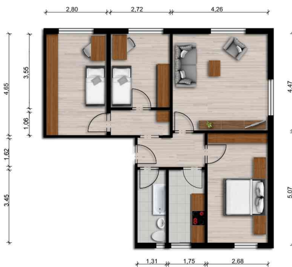
Grundriss
