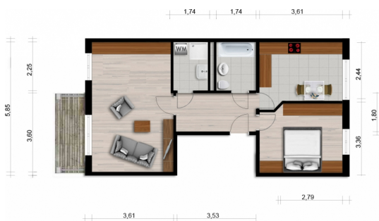
Grundriss
